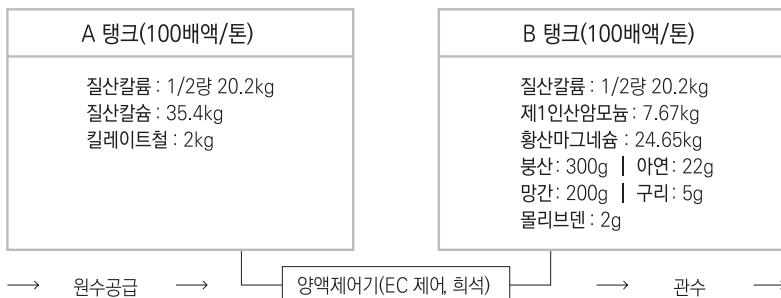
(그림 6-4) 야마자키 배양액에 대한 원액 조제 및 액비혼입 개략도
