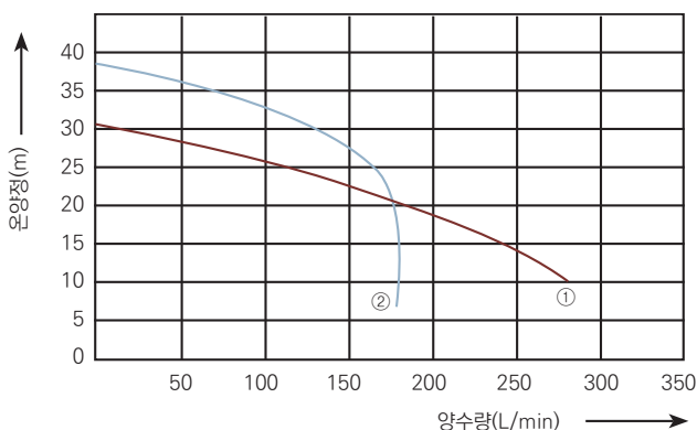
(그림 5-1) 펌프의 온양정에 따른 양수량
