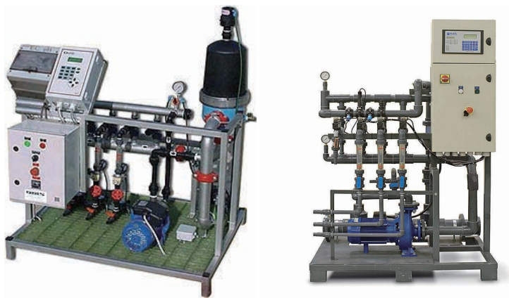
(그림 5-6) 자동관비장치
