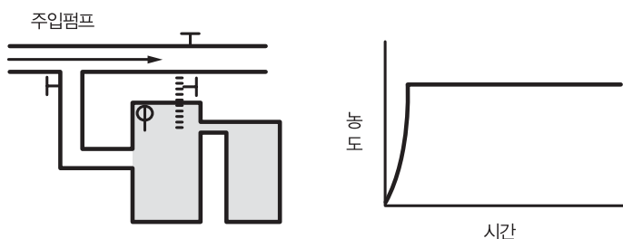
(그림 5-5) 주입 펌프형(Injection Pump Type)
