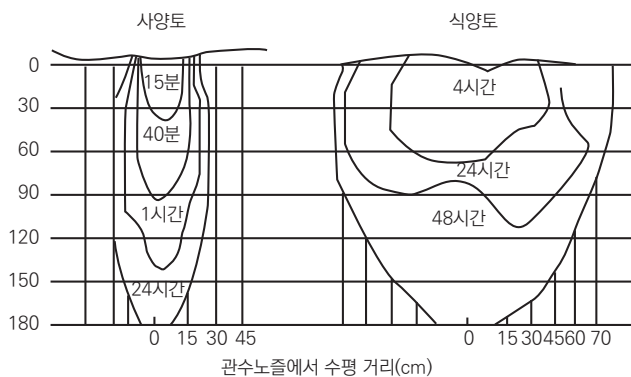
(그림 5-7) 토성에 따른 수분의 이동속도
