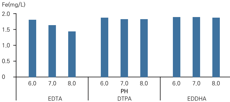
(그림 6-7) 배양액 pH에 따른 킬레이트 Fe의 종류별 불용화 비교(2009, 경남기술원)
