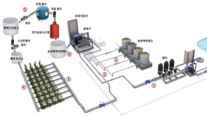
(그림 6-3) 순환식 수경재배 양액의 흐름도
