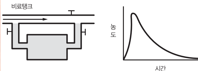
(그림 5-4) 비료 탱크형(Fertilizer Tank Type)
